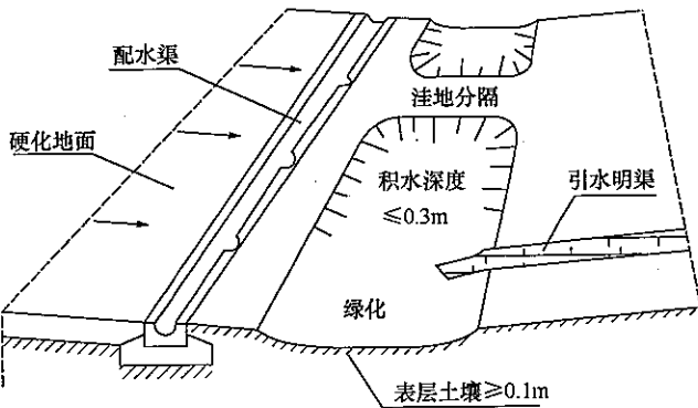
图 11 洼地入渗系统
