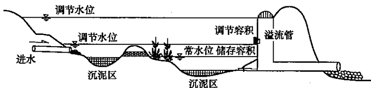
图 22 湿塘
