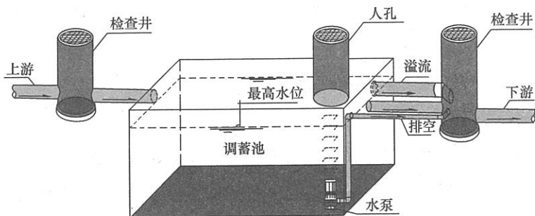
图 23 调蓄池示意
