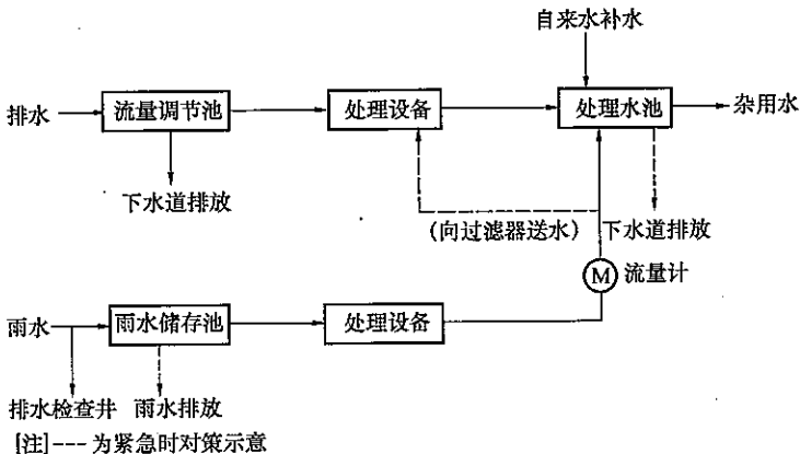
图 2 雨水、中水结合的工艺流程图
