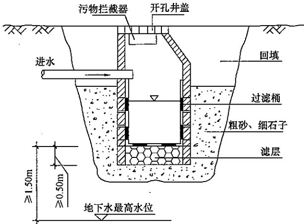
图 15 渗井 A
